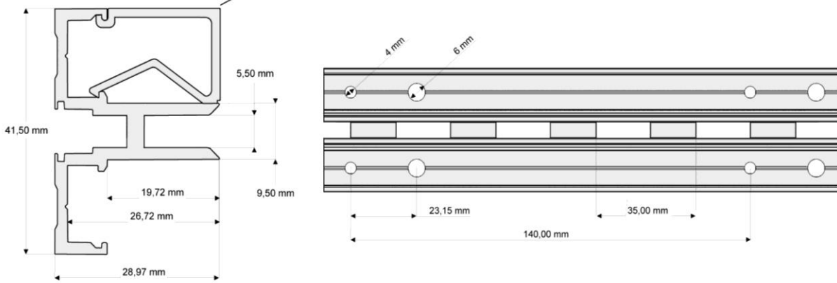
Clipsprofiel / profilé de clips
